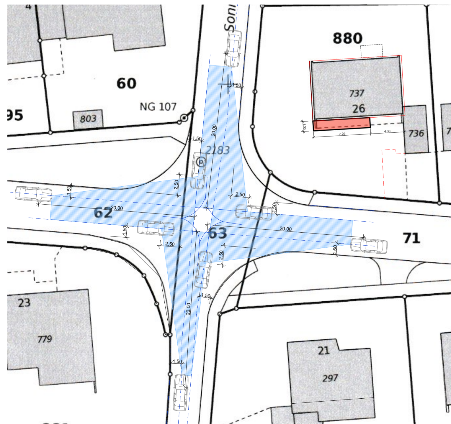
Sichtverhältnisse an Knoten mit Rechtsvortritt
